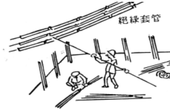
圖三十二、 作業中物體可能接觸之高壓線路應 加裝絕緣套管
