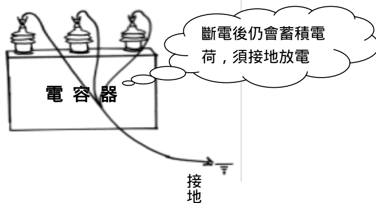
圖二十八、 停電後，電容器仍有殘留電荷，應進行接地放電
