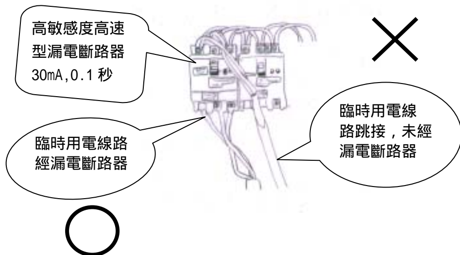
圖七、 電氣線路應確實經過漏電斷路器
