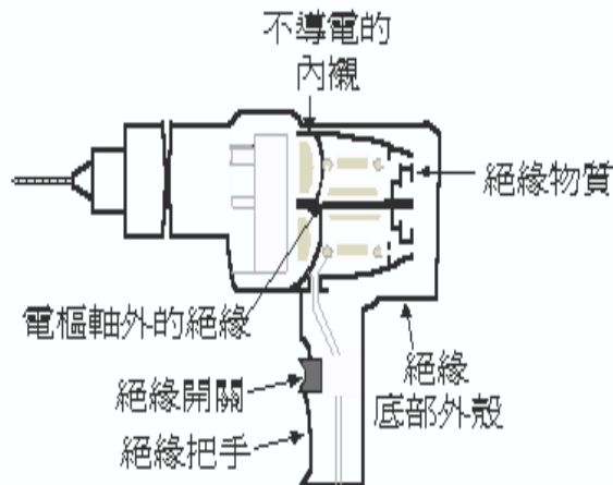
圖九、 電動機具雙重絕緣構造
