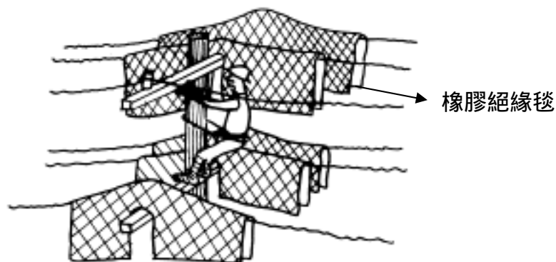
圖三十一、 活線作業勞工身體六十公分內之電路應以絕緣防護
