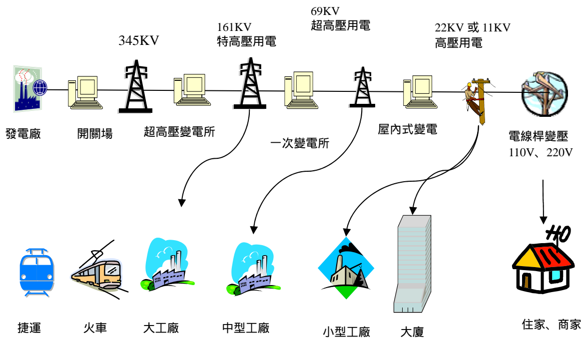
圖一、 電力輸配圖
